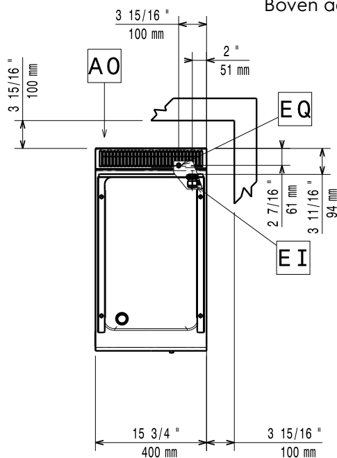
Boven aanzicht
